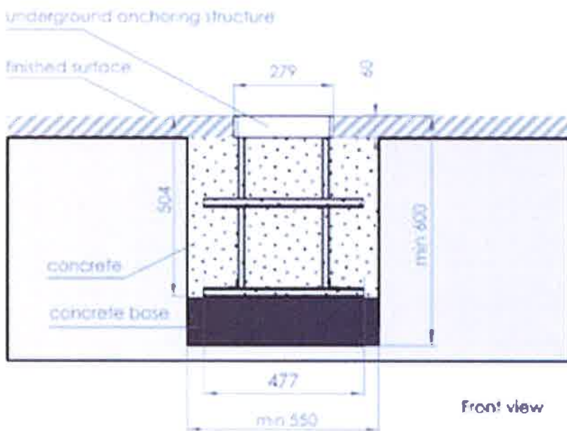
Slika 8: Izvedba osnovne gradbene jame - vzdolžni presek
